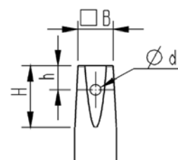
Dimensions stem top:
