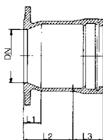
S-9570-4 Flanged socket PN 16
